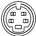
S-VIDEO OUT (female)
